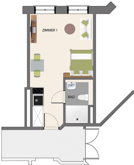
Typ 3: 1 Zimmer, ca. 23 m 2
